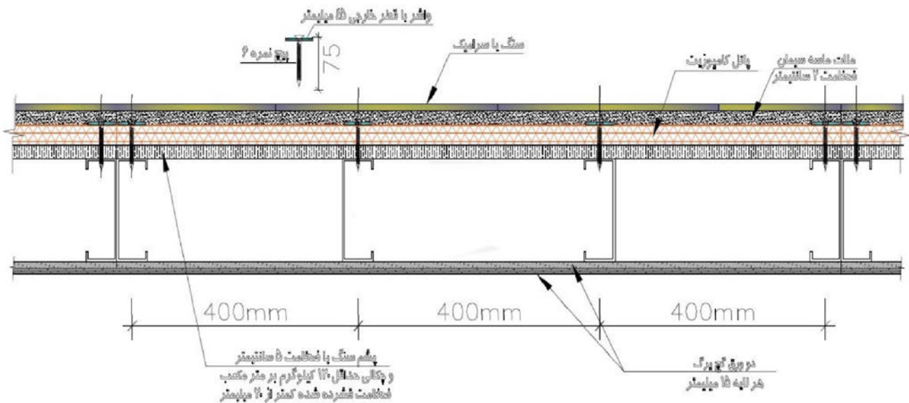
شکل ۱- مقطع سقف سازه‌ای مشتمل بر پانل‌های کامپوزیتی به عرض ۱۲۰ سانتی متر
